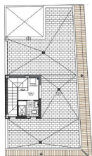
PLANTA SEGUNDA DE 100,00 M 2
